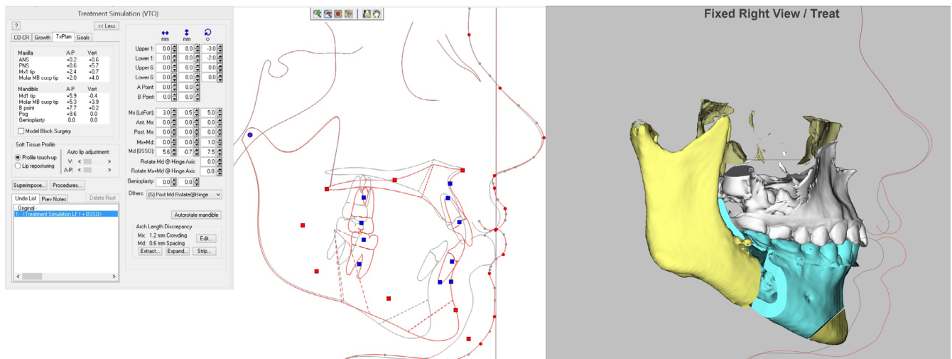
Рис. 1. Схема операции: двусторонняя сагиттальная остеотомия нижней челюсти и остеотомия верхней челюсти на уровне Le Fort I
