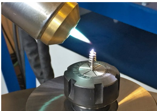
Рис. 1. Нанесение на дентальный имплантат покрытия Pateks [Fig. 1. Process of applying Pateks coating to a dental implant]
